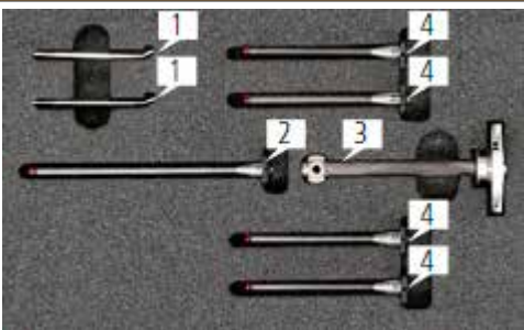
Stylus holder kit TL3, long 형식 : 626103-9058-000
