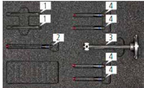
Star stylus kit TL3 형식 : 626103-9033-000
