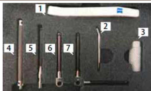
Stylus kit M3 XXT, large star stylus 형식 : 626109-9023-000
